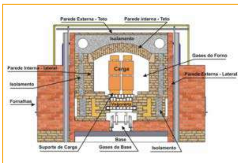
Figuras 27/28 - Representação da seção transversal de um forno túnel e da carga. Fonte: Dadam, 2005 (acima); Dadam e Nicolau, 2006 (abaixo).
