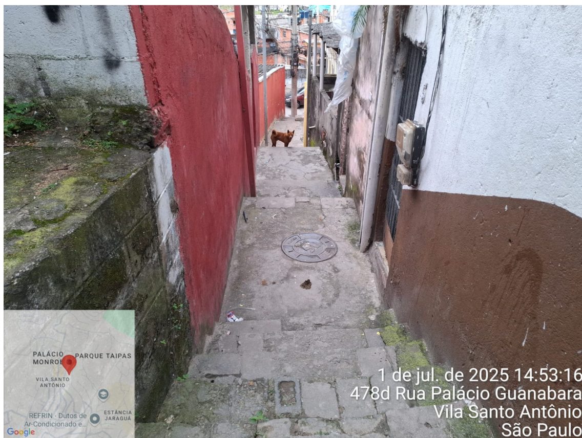
Poço de visita (PV) de esgoto
