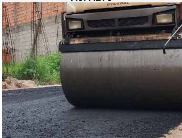
FOTO 18 – COMPACTAÇÃO FINAL
