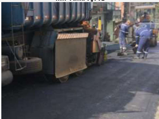
FOTO 15 – TRANSPORTE E APLICAÇÃO DE CAMADA DE ASFALTO
