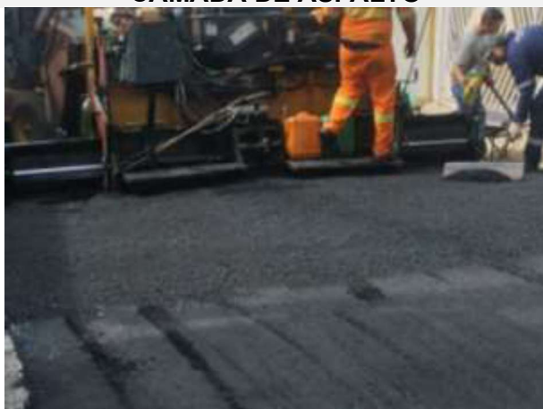
FOTO 17 – EXECUÇÃO DE CAMADA DE ASFALTO
