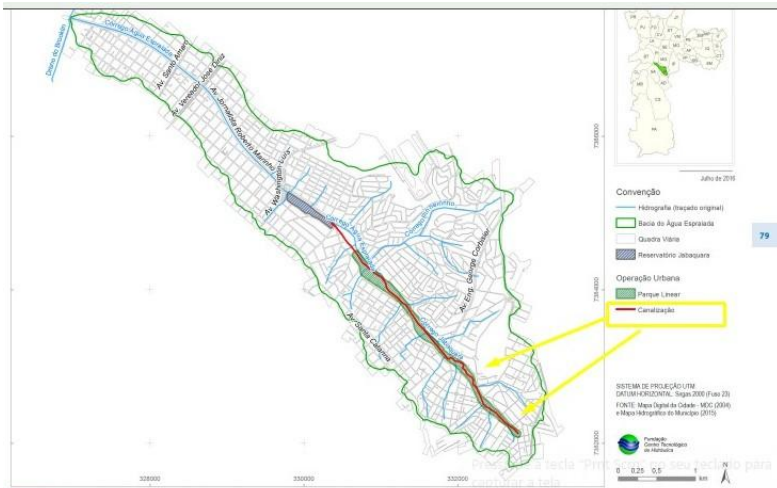
FIGURA 6.1 Infraestrutura proposta para o sistema de drenagem pela Operação Urbana Água Espraiada
